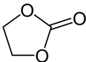
Carbonate d'éthylène
