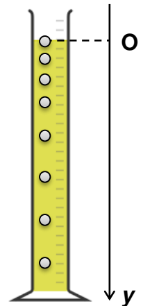
Chronophotographie de la chute de la bille
